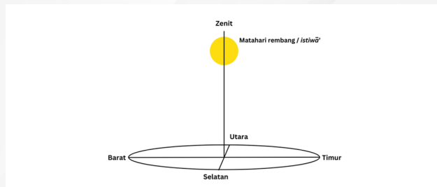
Rajah 1.1 Kedudukan matahari rembang atau istiwa . Pusat matahari berada di meridian tempatan. Sumber: Hardi 2011 [2]
