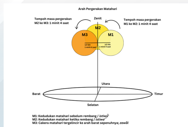
Rajah 1.3 Peralihan matahari dari M1 ke M3
