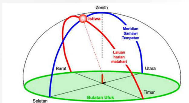
Rajah 1.2 Kedudukan matahari semasa istiwa Sumber: Wan Kamel Wan Hussaid
